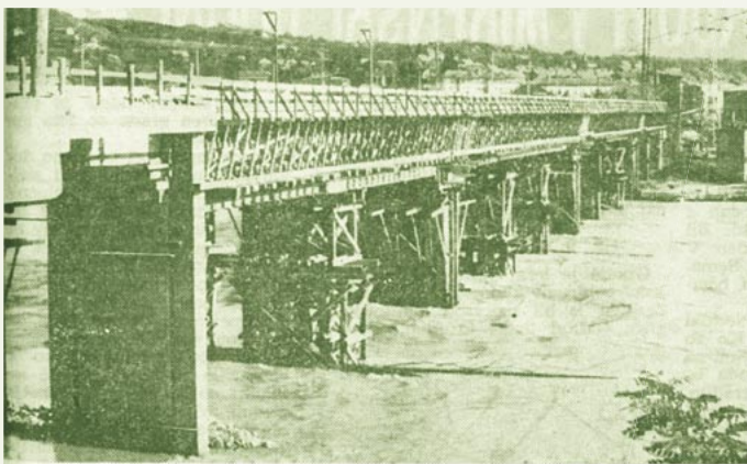
KRSKI MOST V LESENEM OKLEPU. Novi most čez Savo v Krškem je največja gradnja v tej občini. Pretekli teden so delavci PIONIRJA zalili z betonom bodočo vez med obema bregovima Save (Foto: Vili Videnič, drugo mesto za fotografijo tedna, ORWO NP 18, 8, 1/125).
